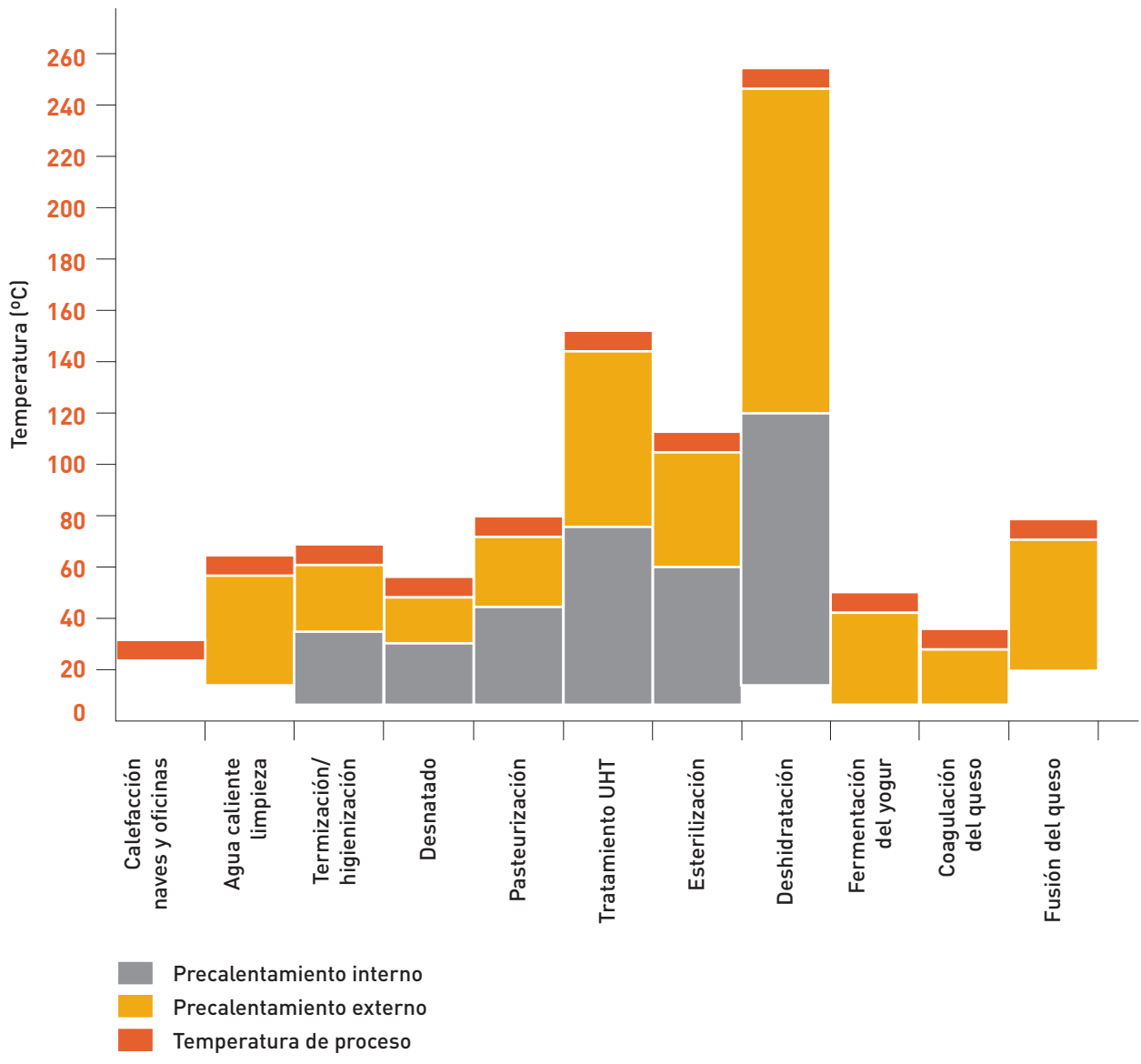
Figura 2.5.2. Procesos consumidores de calor. Niveles de temperatura (temperatura mínima de suministro T_{PS,min} )
