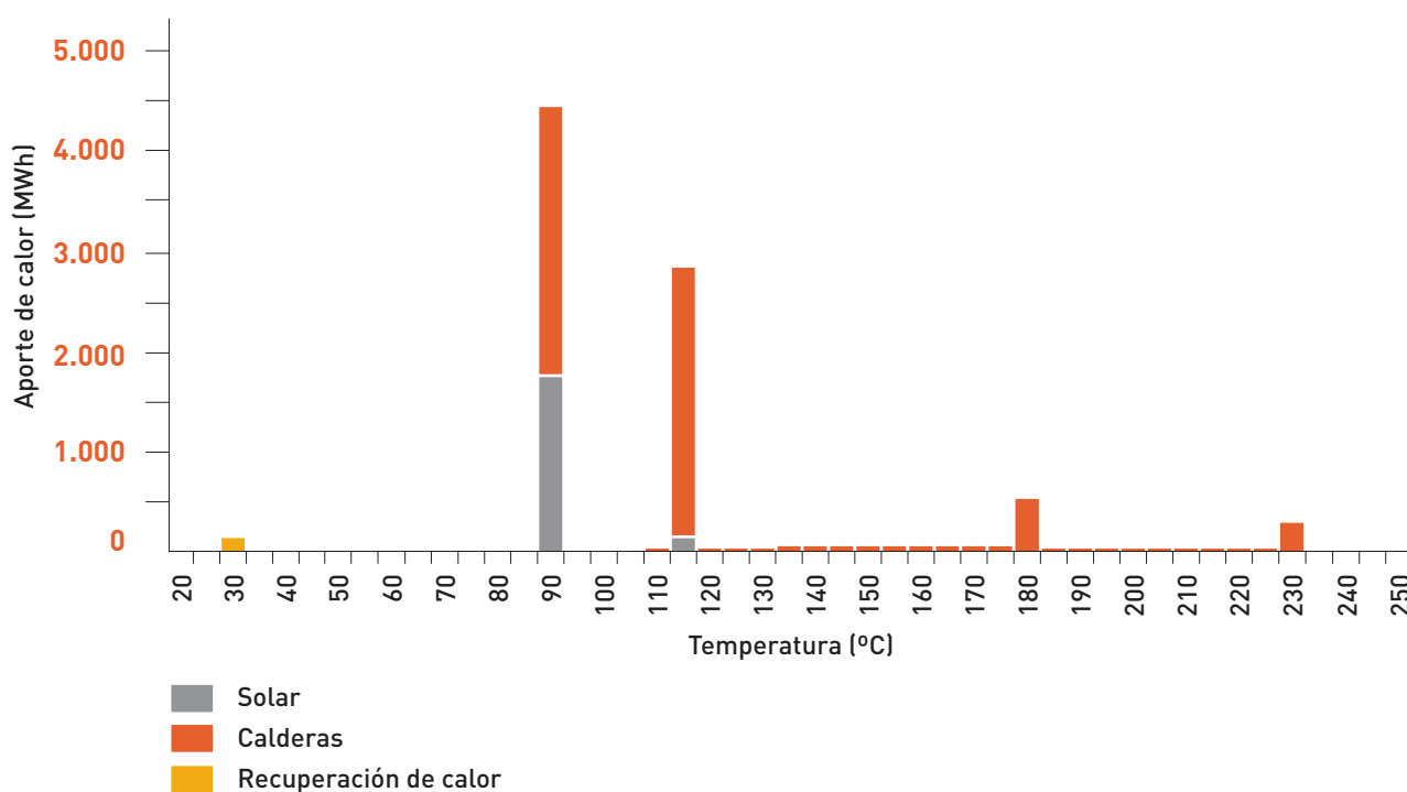
Figura 2.19.6. Aportación de calor sistema solar según niveles de temperatura. Empresa modelo, captadores planos, únicamente para demandas de calor, Zona IV
