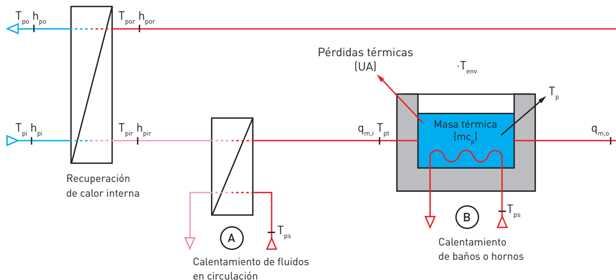
Figura 1.1.1. Modelo de proceso estándar EINSTEIN con un flujo entrante y otro saliente
