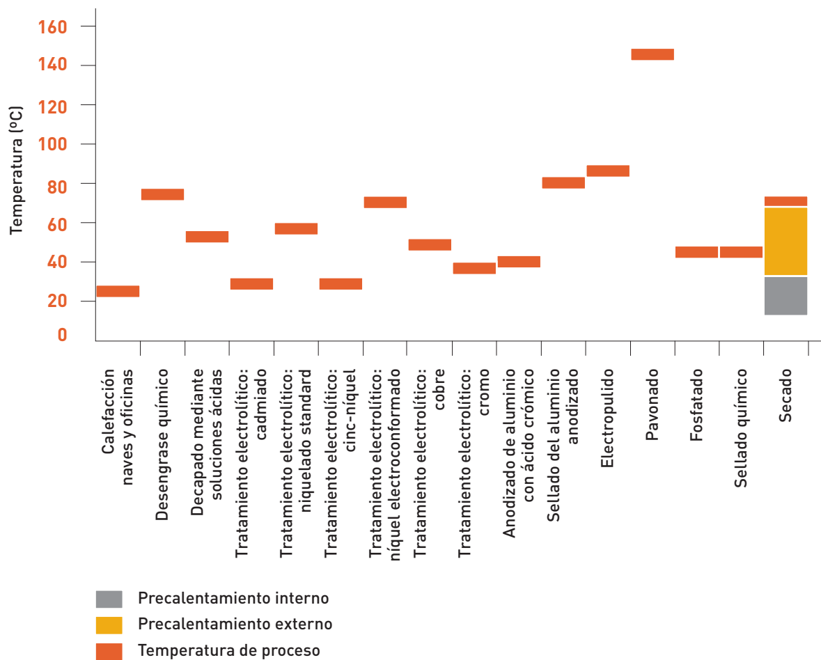
Figura 2.29.2. Procesos consumidores de calor. Niveles de temperatura (temperatura mínima de suministro T_{PS,min} )
