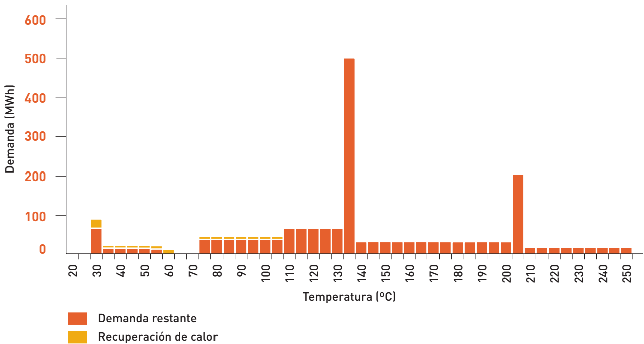
Figura 2.15.3. Consumo de calor según niveles de temperatura. Considerando únicamente procesos consumidores de calor
