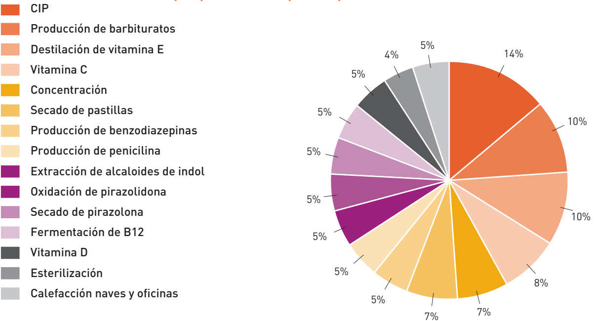
Figura 2.24.1. Consumo de calor por procesos. Empresa tipo del sector
