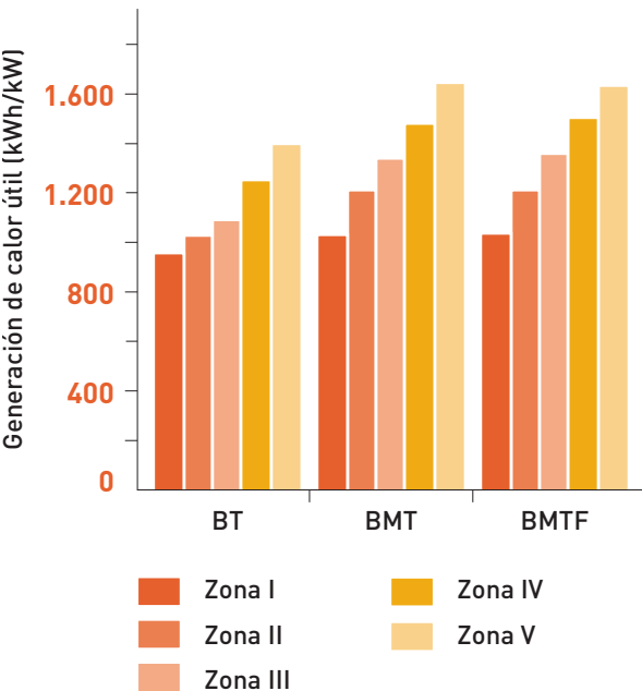
Figura 2.14.9. Generación media de calor útil por unidad de potencia instalada
