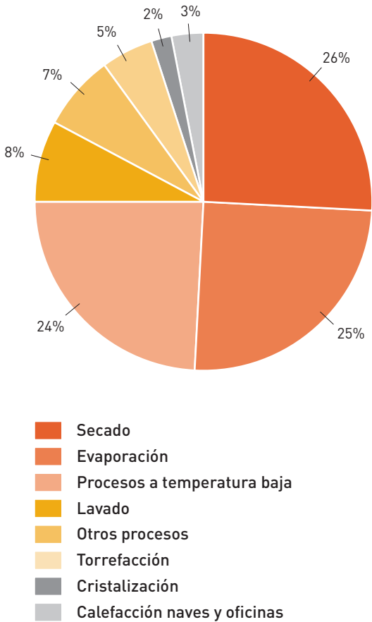
Figura 2.9.1. Consumo de calor por procesos. Empresa tipo del sector
