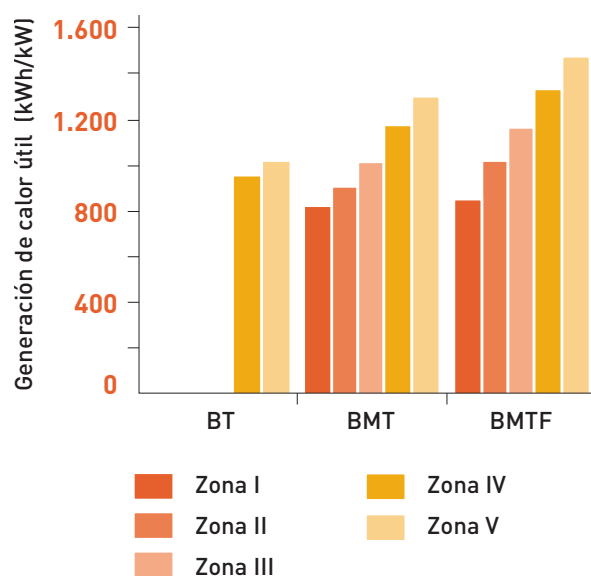
Figura 2.20.10. Generación media de calor útil por unidad de potencia instalada
