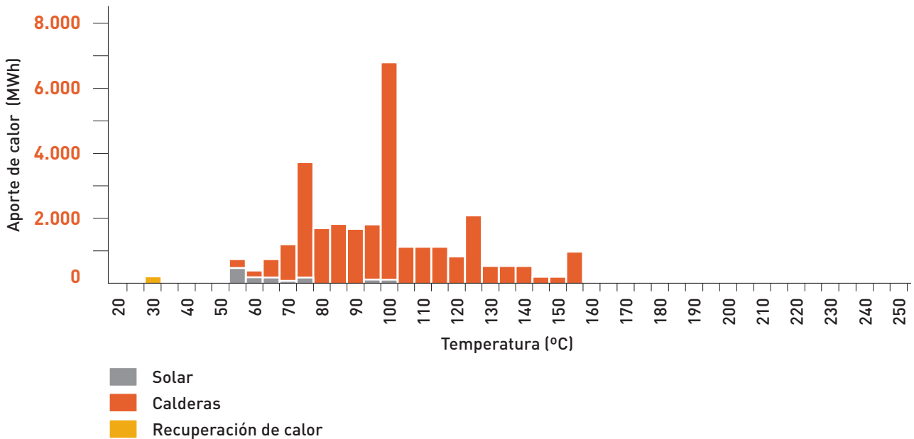
Figura 2.17.7. Aportación de calor sistema solar según niveles de temperatura. Empresa modelo, captadores planos, únicamente para demandas de calor, Zona IV
