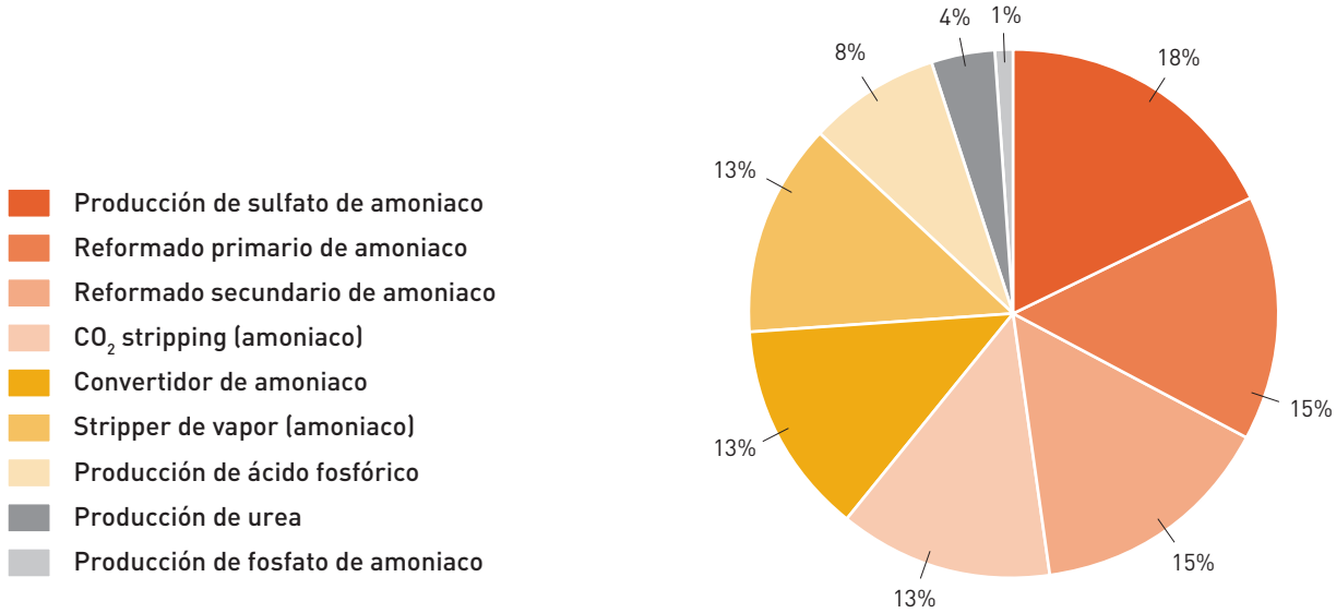
Figura 2.20.1. Consumo de calor por procesos. Empresa tipo del sector
