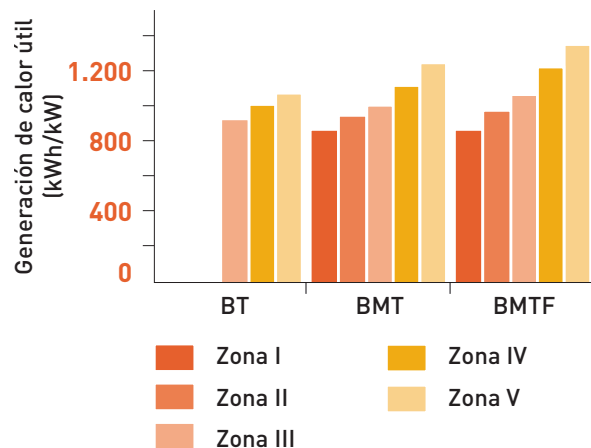
Figura 2.3.10. Generación media de calor útil por unidad de potencia instalada
