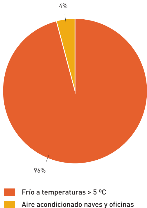
Figura 2.19.3. Consumo de calor equivalente para consumos de frío. Empresa tipo del sector
