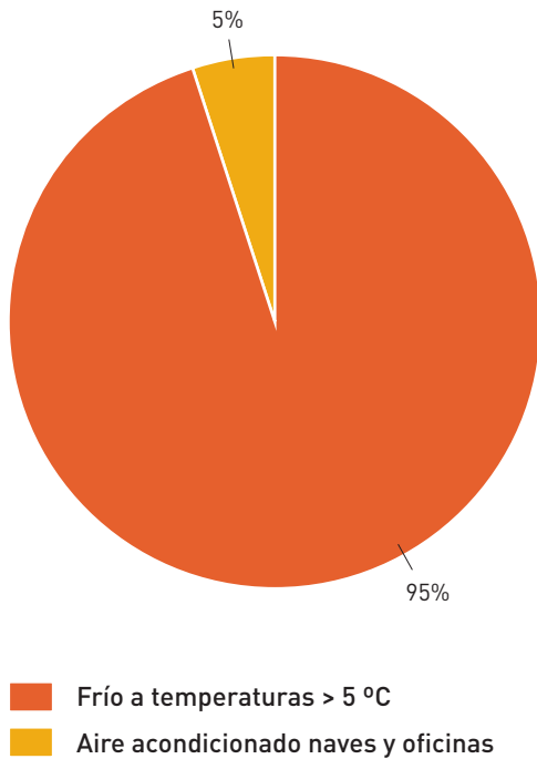
Figura 2.22.3. Consumo de calor equivalente para consumos de frío. Empresa tipo del sector
