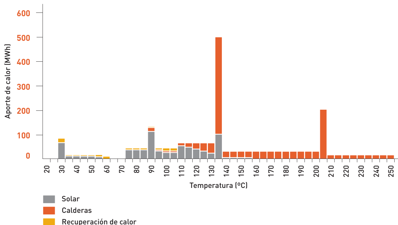
Figura 2.15.6. Aportación de calor sistema solar según niveles de temperatura. Empresa modelo, captadores planos, sólo demandas de calor, Zona IV
