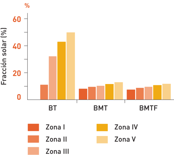
Figura 2.22.8. Fracción solar media del sector
