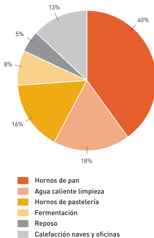
Figura 2.8.1. Consumo de calor por procesos. Empresa tipo del sector
