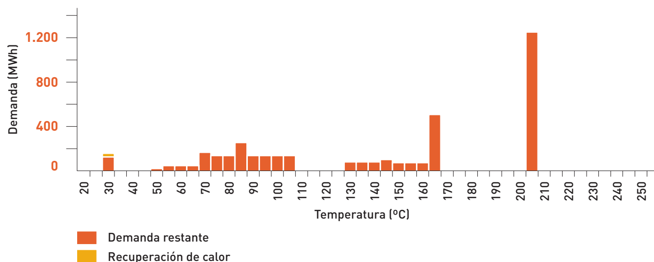
Figura 2.26.3. Consumo de calor según niveles de temperatura. Considerando únicamente procesos consumidores de calor
