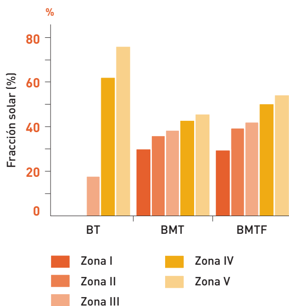
Figura 2.32.7. Fracción solar media del sector
