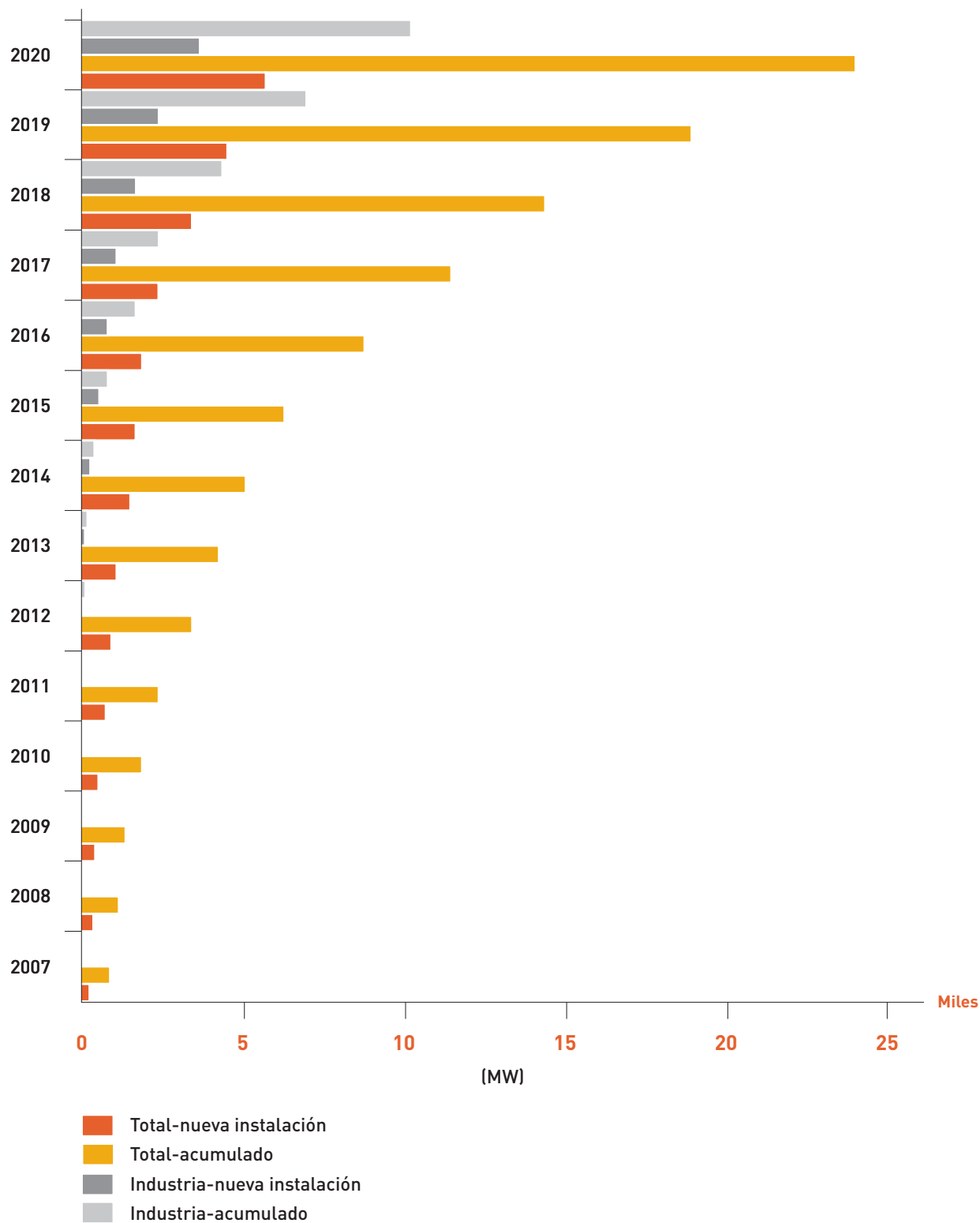
Figura 3.3.4. Posible escenario de la evolución de las instalaciones de energía solar térmica en España y de la contribución de instalaciones industriales según escenario F: tasa de crecimiento general: 30%
