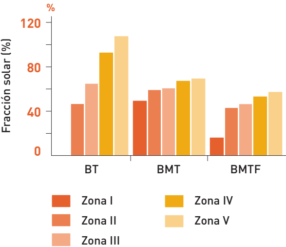
Figura 2.24.8. Fracción solar media del sector
