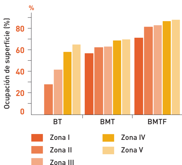
Figura 2.1.9. Grado medio de ocupación de superficie
