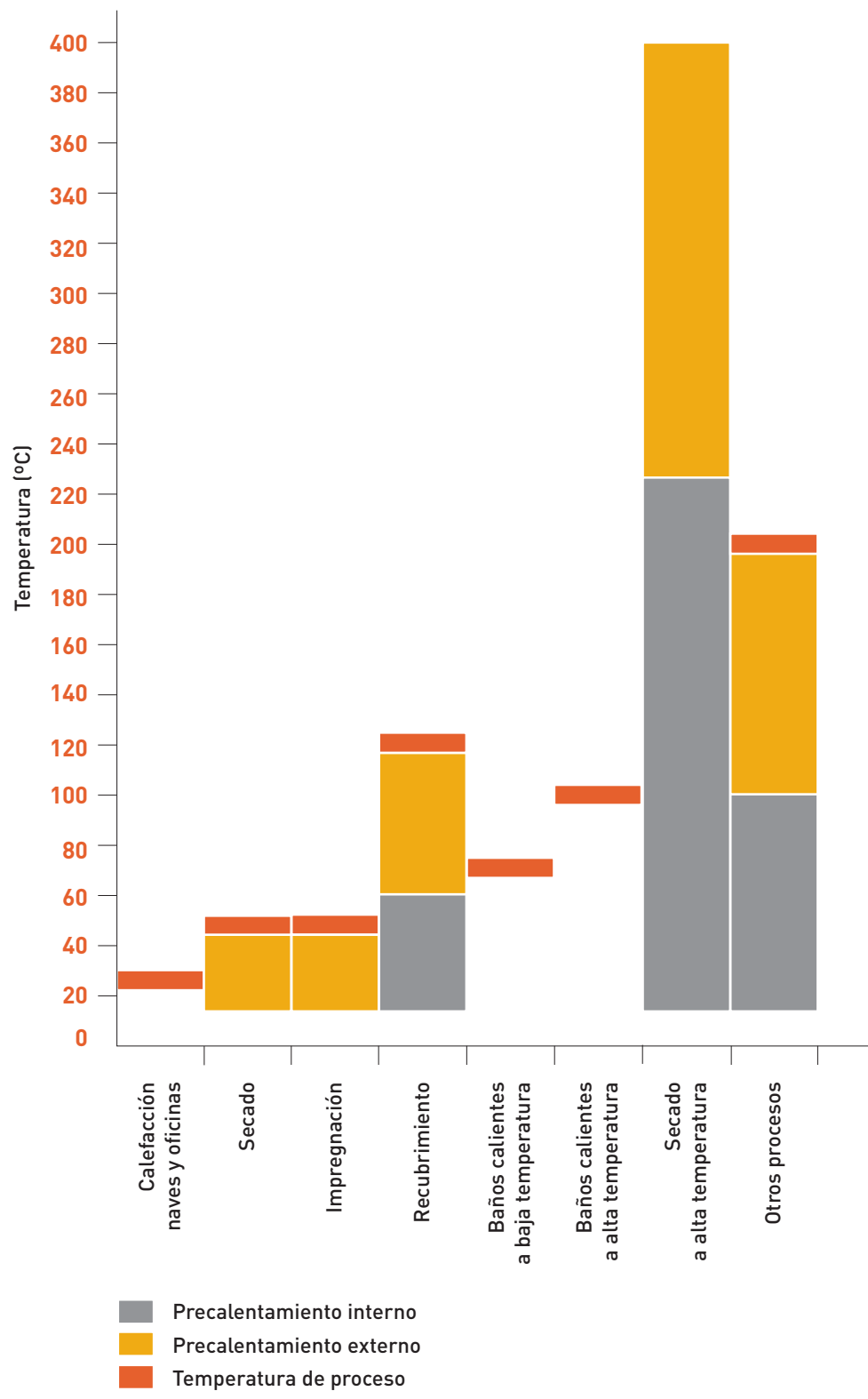
Figura 2.13.2. Procesos consumidores de calor. Niveles de temperatura (temperatura mínima de suministro T_{PS,min} )
