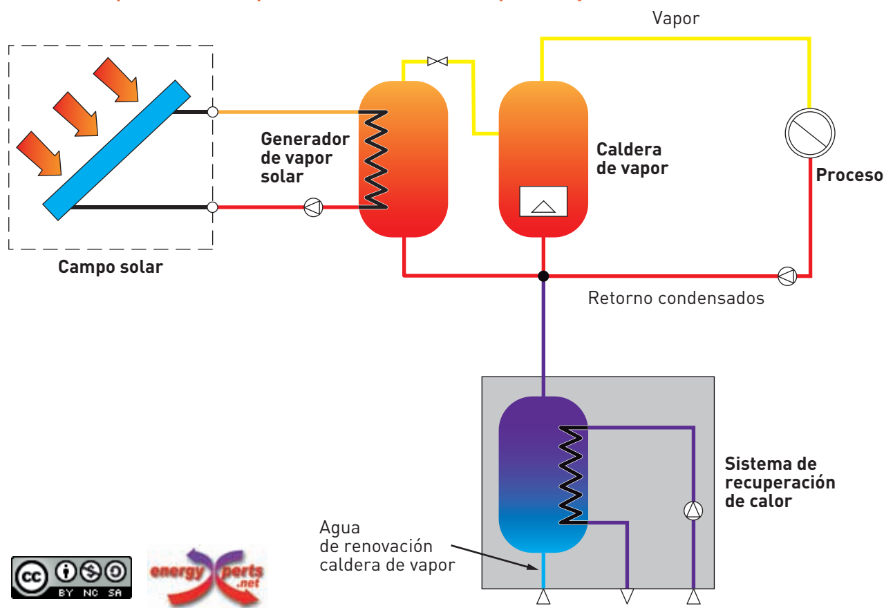
Figura 25. Esquema del principio de funcionamiento de un sistema solar térmico para la generación directa de vapor. Sistema VDPac con caldera auxiliar en paralelo y acumulación de calor
