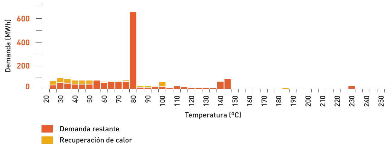
Figura 2.4.3. Consumo de calor según niveles de temperatura. Considerando únicamente procesos consumidores de calor
