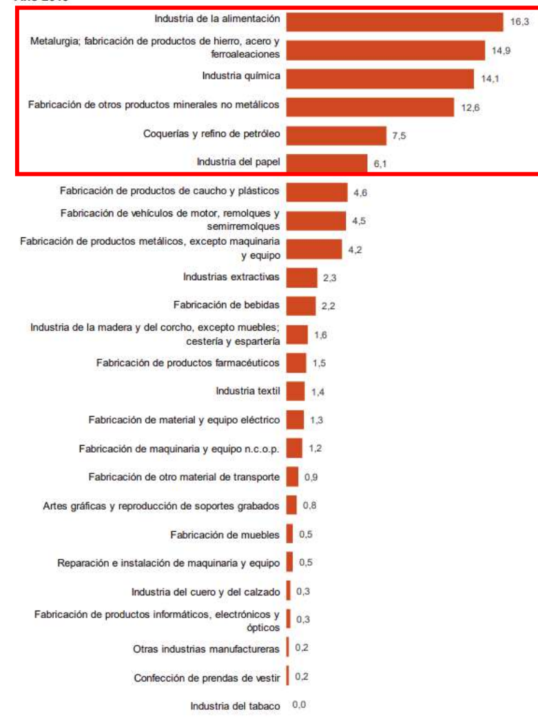
Distribución porcentual del consumo energético en la industria, por ramas de actividad. Año 2019
